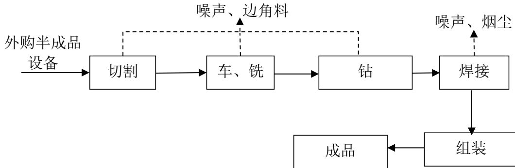
图 2 项目工艺流程与产污环节图
