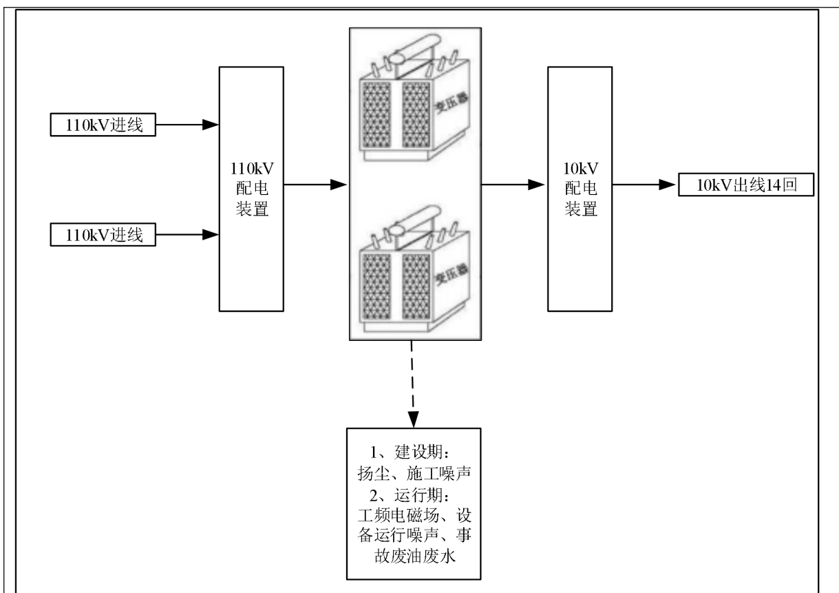
图 4-3 110kV 变电站工艺流程及环境影响示意图
