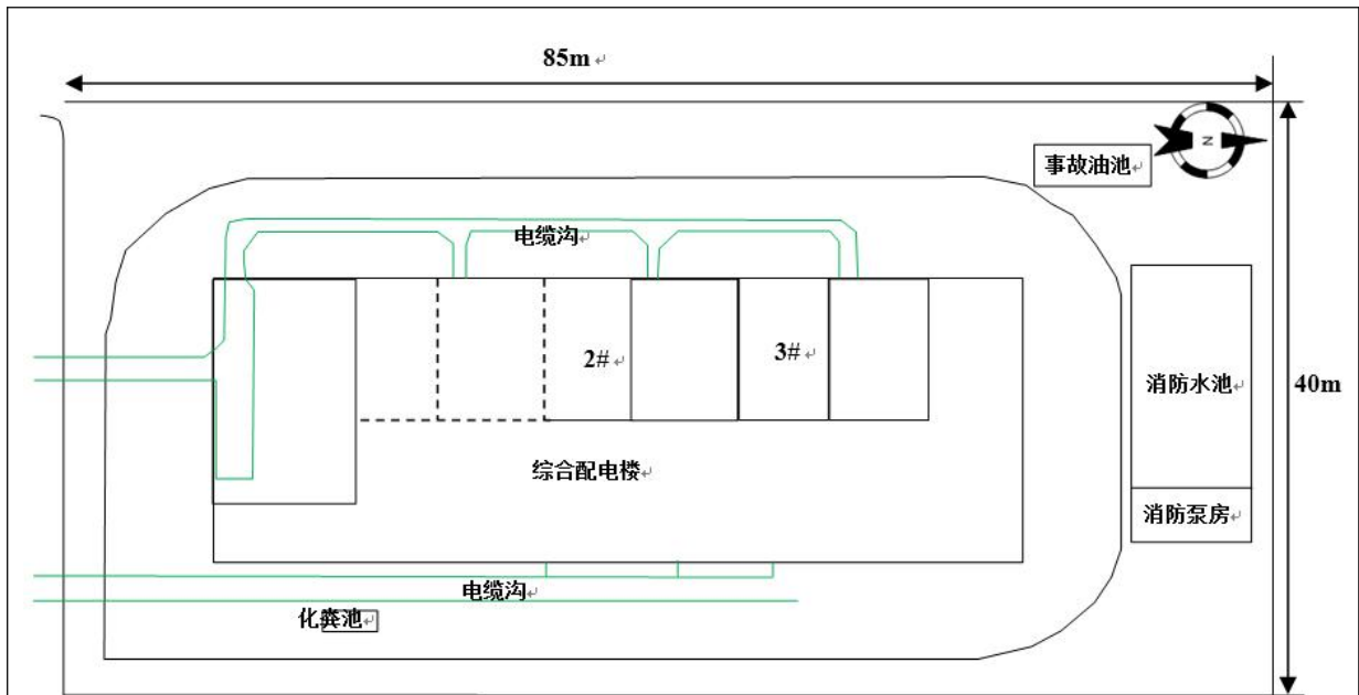
图 4-2 兴咸 110kV 变电站总平面布置图
