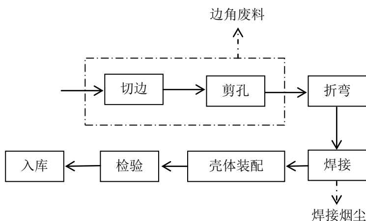
图 2 项目工艺流程与产污环节图
