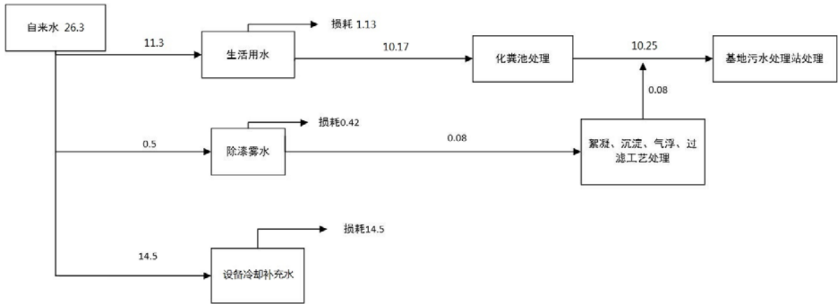
图 3.3-1 项目水平衡图
