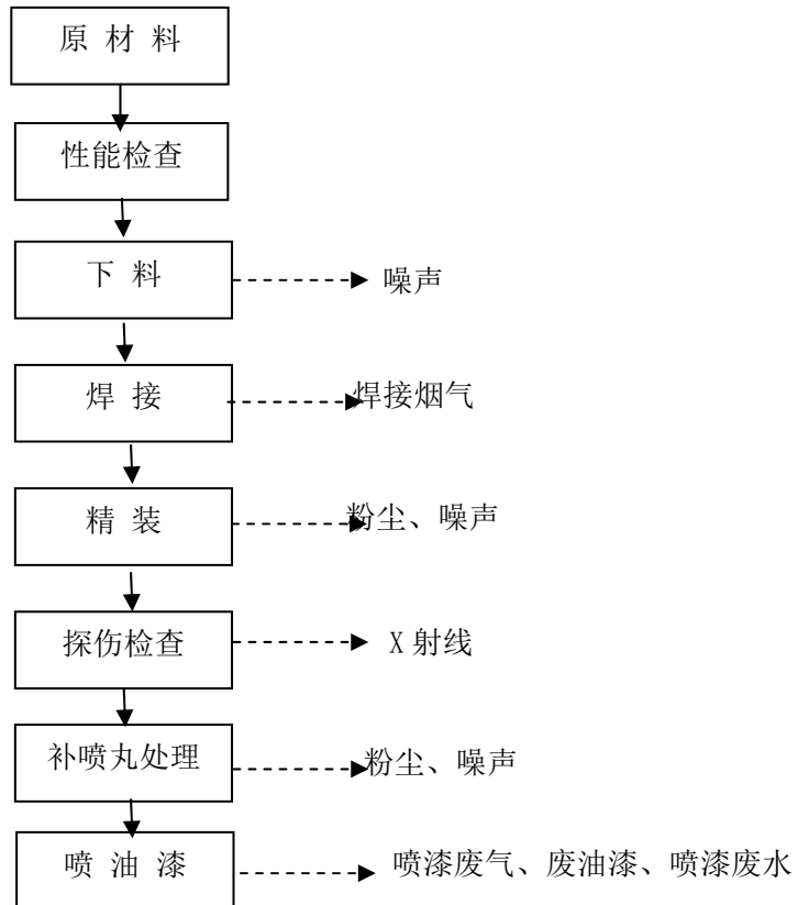
图 3.4-1 钢桥产品生产工艺流程以及产污环节图
